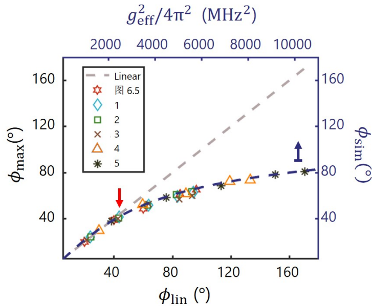
图 6.7 集体微波响应由线性转为非线性的现象。其中， \phi_{lin} = \sum_k \phi_k 为各个 DQD 最大微波相位响应之和。灰色的虚线为线性估计下的集体微波响应，它满足公式 \phi_{max} = \phi_{lin} 。深蓝色的虚线模拟了一个耦合到谐振腔上的激发子在不同耦合强度 g_{eff} 下对谐振腔相位 \phi_{sim} 的影响。它的频率为 \omega_{eff}/2\pi = 5.7 GHz，退相干速率为 \gamma_{eff}/2\pi = 50 MHz。相位移动 \phi_{sim} 是根据公式 S_{21} = \frac{A_0}{g_{eff}\chi_{eff} + \kappa/2} 计算得出的。从图中我们可以看出，线性近似在 \phi_{lin} \sim 45^\circ 或 (g_{eff}/2\pi)^2 = 55^2 \text{ MHz}^2 (这两个位置满足 \sum_k g_k \chi_k = g_{eff}\chi_{eff} \sim \kappa/2 ) 开始与实验现象明显不符。
