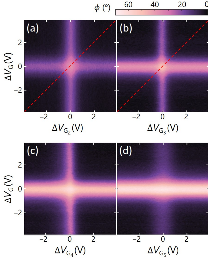
图 6.5 多比特关联谱，谐振腔的相位响应 \phi 与 \Delta V_{G_k} 和 \Delta V_G 之间的关系图。(a) \text{DQD}_1 与 \text{DQD}_2 之间的两比特关联谱。此处， \Delta V_G = \Delta V_{G_1} 。(b) - (d) 展示了多比特关联谱。 \text{DQD}_3 、 \text{DQD}_4 、 \text{DQD}_5 依次被添加进来。其中， G 为上一张图中所有使用过的电极的集合。在 (b) 中， G = \{G_1, G_2\} 。在 (c) 中， G = \{G_1, G_2, G_3\} 。在 (d) 中， G = \{G_1, G_2, G_3, G_4\} 。
