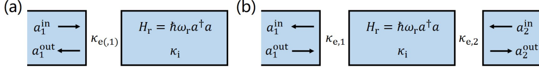
图 2.7 谐振腔端口网络示意图。(a) 单端口反射式谐振腔。(b) 双端口透射式谐振腔。
