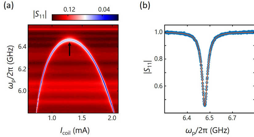
图 5.2 (a) SQUID 阵列谐振腔的谐振频率 \omega_r 随通过磁线圈中的电流 I_{\text{coil}} 的变化关系。(b) 谐振腔反射谱。谐振腔的反射率 |S_{11}| 随着探测频率 \omega_p/2\pi 的变化而变化，谐振腔的谐振频率为 \omega_r/2\pi = 6.48 GHz。图中蓝色的圆圈为实验数据，红色的曲线为拟合得到的曲线。该数据已经扣除了本底信号。
