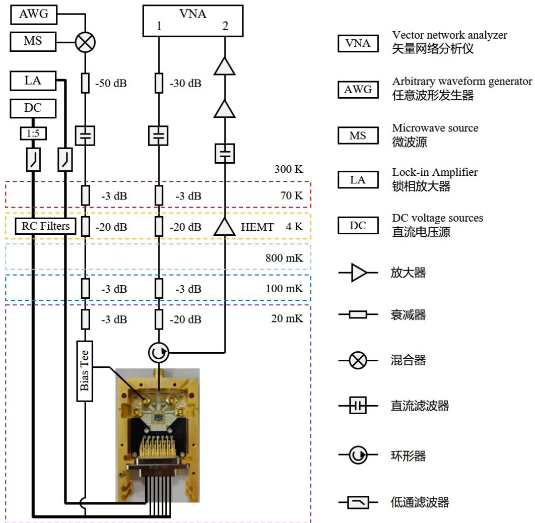
图 5 测控线路总览。
