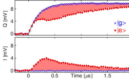
图 4.2 利用主方程模拟得到的测量信号轨迹与实验数据的对比图。图片自于 [21]。
