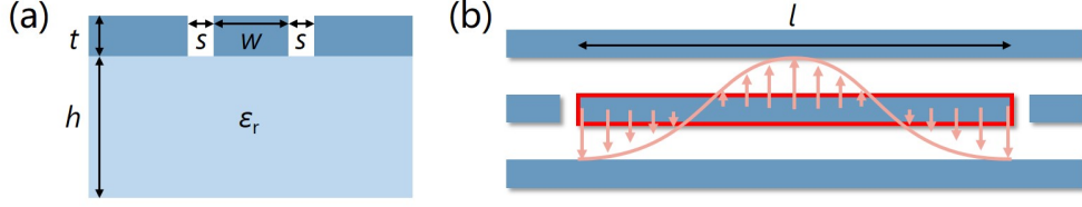
图 2.6 共面波导谐振腔示意图。(a) 共面波导传输线的横截面示意图。其中，中心导体宽度为 w ，中心导体与两侧地平面的间隔为 s ，膜的厚度为 t 。而在共面波导传输线结构下方的基片厚度为 h ，相对介电常数为 \varepsilon_r 。(b) 共面波导透射腔结构的示意图。中间由红色方框所示的为透射腔部分，与两端的传输线存在电容耦合。电磁场在谐振腔内形成驻波，图中使用粉红色标图图形为谐振腔内产生的全波长驻波示意图。
