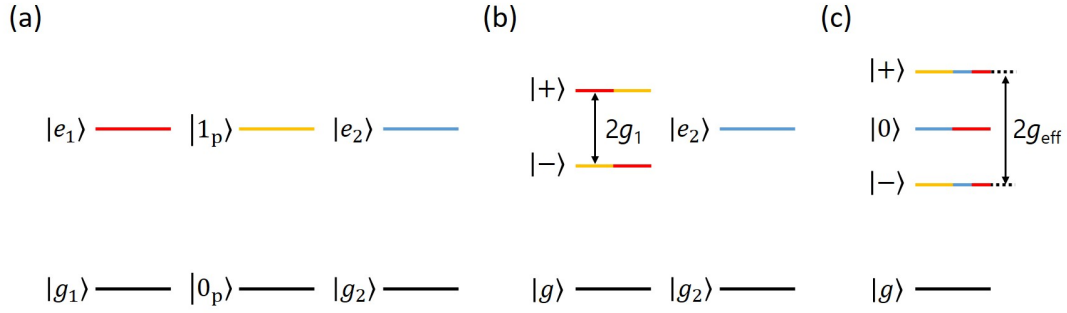
图 5.6 Tavis-Cummings 模型能级示意图 ( \omega_{a,1} = \omega_{a,2} = \omega_r ), 取 \hbar = 1 。(a) 三个子系统不存在相互作用时的能级示意图。(b) 仅比特 1 与谐振腔存在相互作用时 (Janes-Cummings 模型) 的能级示意图。(c) 比特 1 与比特 2 都与谐振腔存在相互作用时的能级示意图。图中不同态成分通过颜色进行标记。耦合后形成的本征态通过不同颜色、不同长短的线段展示该态中拥有的成分以及对应成分所占的比例。
