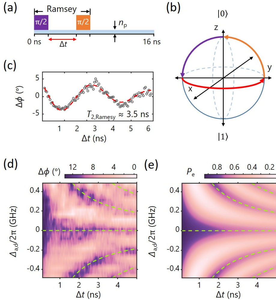
图 4.4 利用时间平均色散读出法表征 Ramsey 干涉。(a) Ramsey 干涉脉冲序列示意图。其中用于实现 Ramsey 操作的微波序列有两个间隔时间为 \Delta t 、频率为 \omega_d 的 \pi/2 操作构成。用于测量谐振腔相位响应的探测微波频率为 \omega_p/2\pi = \omega_t/2\pi = 6.53\text{GHz} 。(b) 利用 Bloch 球表现 Ramsey 干涉过程。(c) 测量时间平均相位响应信号 \Delta\phi 与间隔时间 \Delta t 的关系图。此时，比特频率与驱动微波频率的差值为 \Delta_{a,d}/2\pi = -375\text{MHz} ，间隔时间为 \Delta t = 0.75\text{ns} 。灰色的圆圈为实验数据，虚线为拟合曲线。(d) Ramsey 振荡速率与 \Delta_{a,d} 的关系图。(e) 模拟 Ramsey 振荡速率与 \Delta_{a,d} 的关系图，模拟参数为 T_{2,\text{Ramsey}} = 3.5\text{ns} 。 P_e 为比特激发态的占据概率。
