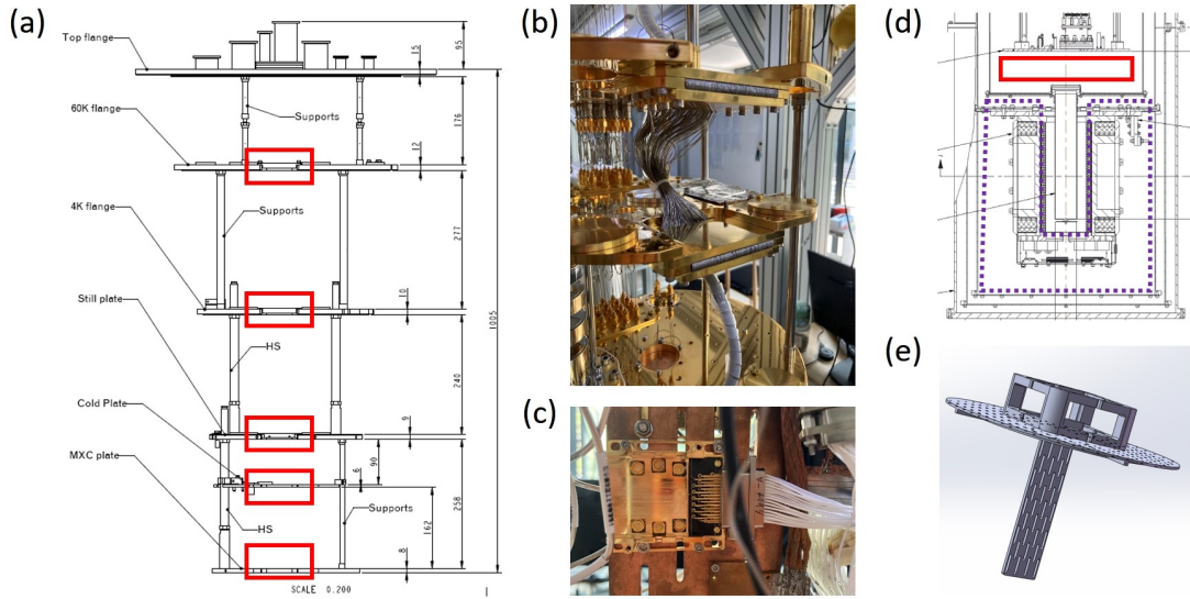
图 4 (a) 稀释制冷机内部结构示意图。该型号为 LD-250，生产公司为 Bluefors。(b) 在稀释制冷机上加装的直连线组。通过热沉夹板与稀释制冷机中的每一层都形成了良好的热接触。(c) 通过冷指安装在混合腔层的样品盒。(d) 加装了磁体的稀释制冷机结构示意图。红框部分为我们想通过加装额外平台利用的稀释制冷机的内部空间，紫色部分为加装磁体会占用的空间。(e) 加装的额外平台部分示意图。从上到下依次为支撑连接部、额外盘面以及冷指。
