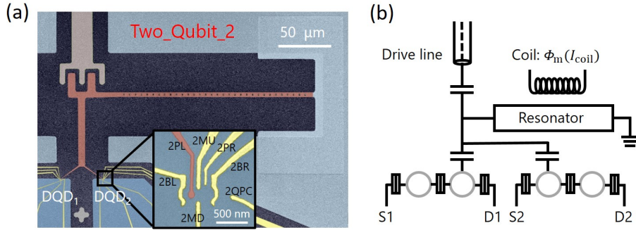
图 3.2 微波谐振腔与半导体量子点集成芯片的。该样品为 Two_Qubit_2。(a) 样品在光镜下拍摄的照片（伪色）。其中，米色部分为传输线，红色部分为 SQUID 阵列谐振腔，黄色部分为两个双量子点使用的金属电极，淡蓝色部分为谐振腔的地平面。其中，内插图右侧量子点的局部放大图，是通过扫描电子显微镜照片拍摄的（伪色）。(b) 样品电路示意图。其中，谐振腔的频率通过悬挂在样品盒上的磁线圈控制。我们通过改变通过磁线圈内部的电流大小 I_{\text{coil}} 来调节通过 SQUID 的磁通大小 \Phi_m 。
