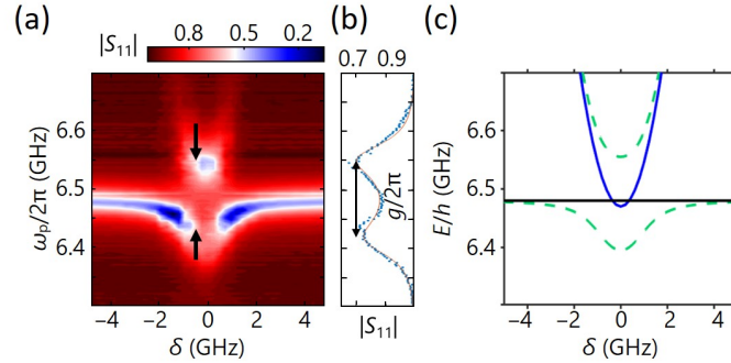
图 3.7 真空 Rabi 劈裂。数据来自与样品 Two_Qubit_2 中左侧的双量子点。(a) 受电荷比特调制的谐振腔频谱图。在黑色箭头位置处，比特频率与谐振腔频率相等并发生真空 Rabi 劈裂，产生了两条劈裂宽度为 2g/2\pi = 2 \times 81 MHz 的谱线。(b) 在图 (a) 黑色箭头处截取得到的谐振腔频谱图。图中的红色实线为式3.1的拟合曲线。我们注意到，在比特与光子共振时，它们形成了最大杂化态，两条谱线对应的线宽一致，为比特线宽和谐振腔线宽的算术平均值 [1,20-21] 。(c) 利用 J-C 模型模拟的杂化系统能级图。其中黑色实线与蓝色实线分别为未发生耦合时光子与比特的能级，而绿色虚线为发生耦合后杂化系统的能级。模式所用到的参数为隧穿速率 2t/2\pi = 6.47 GHz、谐振腔频率 \omega_r = 6.48 GHz、电荷比特与光子的耦合强度为 g/2\pi = 81 MHz。
