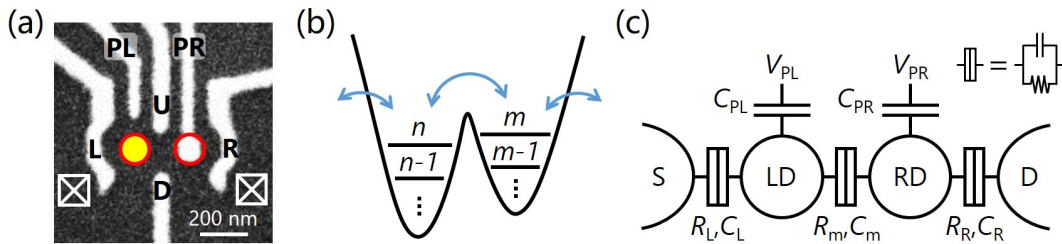
图 2.2 门控双量子点。 (a) 门控双量子点的扫描电子显微镜照片。红圈表示两个量子点的形成位置。(b) 双量子点的束缚势示意图。在两侧势阱中都存在数个分立的能级，电子可越过中间的势垒在两个量子点之间跃迁。同时，电子也可以在源漏电子库以及量子点之间跃迁。(c) 双量子点的等效电路图。电子处于左量子点 (LD) 以及右量子点 (RD) 之中。两侧源漏电子库分标记为 S 和 D。其中，隧穿势垒由电阻与电容并联构成，其电容大小受对应电极上的偏置电压控制。
