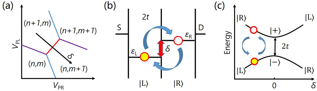
图 2.4 电荷量子比特。(a) 电荷稳态分布示意图。该图为2.3(c)的局部放大图。在图中红线所示处，量子点间的失谐量为0，电子持续地在左点与右点之间进行跃迁。(b) 双量子点内电子跃迁示意图。 2t 为双量子点中电子的点间隧穿速率。 \delta 是双量子点之间的失谐量，为左右量子点电化学势之差 \epsilon_L - \epsilon_R 。(c) 双量子点电荷态能级图。二能级的能量以及成分随着失谐量 \delta 的改变发生变化。
