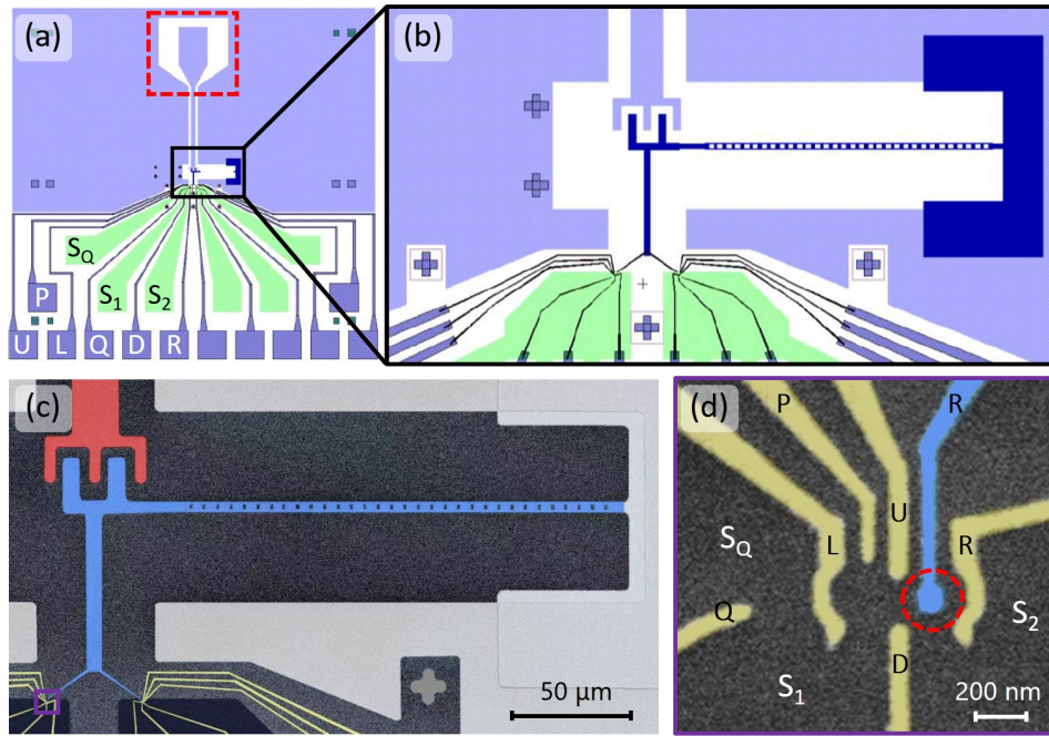
图 1 微波谐振腔与半导体量子点集成芯片的结构示意图。(a) 高阻抗 SQUID 阵列谐振腔与两个双量子点耦合样品的结构设计图。该芯片的整体尺寸为 3 \times 3 \text{ mm}^2 。在该图中，我们标记了左侧量子点使用的电极。其中，电极 P、U、L、D、R 用于控制双量子点性质（节 2.1.2）；电极 Q 被用于量子点接触（quantum point contact, QPC）；电极 S 1 与 S 2 为量子点的源漏电极；电极 S Q 配合 S 1 可以用于测量量子点接触的电流。(b) 为图 (a) 中谐振腔区域的放大图。深蓝色部分从左到右可以分为三个结构，即用于耦合两个量子点以及外部传输线的电极结构、提供高电感的 SQUID 阵列、用于形成地平面的大电容结构。(c) 高阻抗 SQUID 阵列谐振腔与两个双量子点耦合样品的扫描电子显微镜照片（伪色）。其中，红色部分为传输线，蓝色部分为 SQUID 阵列谐振腔，黄色部分为两个双量子点使用的金属电极，银色部分为谐振腔的地平面。由紫色方框圈中的部分为左侧的双量子点。(d) 左侧双量子点的扫描电子显微镜照片（伪色）。
