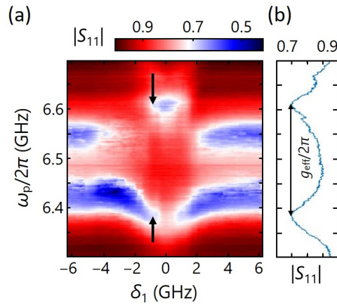
图 5.8 增强真空 Rabi 劈裂。(a) 谐振腔的幅值响应 |S_{11}| 与失谐量 \delta_1 以及探测频率 \omega_p 的关系图。在黑色箭头位置处，发生了增强真空 Rabi 劈裂，产生了两条劈裂宽度为 2g_{\text{eff}}/2\pi = 2 \times 112 MHz 的谱线。参数 \delta_1 的扫描方向为从大到小。在 \delta_1 \sim -3 GHz 附近，比特 2 的频率发生了抖动，因此图像不再中心对称。(b) 在图 (a) 黑色箭头处截取得到的谐振腔频谱图。
