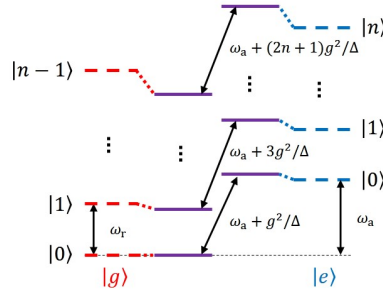
图 2.14 二能级原子与谐振腔大失谐时，Jaynes-Cummings 哈密顿量的能级示意图。红色(蓝色)虚线代表两子系统不存在耦合时，二能级处于基态 |g\rangle(|e\rangle) 且光子数态为 |k\rangle 时的系统能级。紫色实线代表在相互作用下形成的新本征能级。
