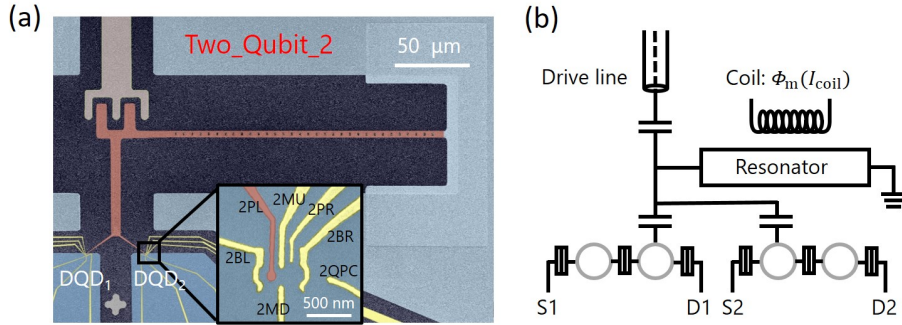
图 5.1 微波谐振腔与半导体量子点集成芯片的结构示意图，编号 Two_Qubit_2。(a) 样品在光镜下拍摄的照片（伪色）。其中，米色部分为传输线，红色部分为高阻抗 SQUID 阵列谐振腔，黄色部分为两个双量子点使用的金属电极，淡蓝色部分为谐振腔的地平面。其中，内插图为右侧量子点的局部放大图，是通过扫描电子显微镜照片拍摄的（伪色）。(b) 样品电路示意图。其中，谐振腔的频率通过悬挂在样品盒上的磁线圈控制。我们通过改变通过磁线圈内部的电流大小 I_{coil} 来调节通过 SQUID 的磁通大小 \Phi_m 。
