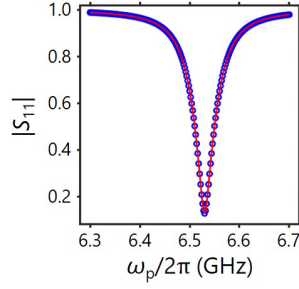
图 3.3 谐振腔反射谱。谐振腔的反射率 |S_{11}| 随着探测频率 \omega_p/2\pi 的变化而变化，并在谐振腔（共振）频率 \omega_r/2\pi = 6.53 GHz 处达到最小值。图中蓝色的圆圈为实验数据，红色的曲线为拟合得到的曲线。该数据已经扣除了本底信号。
